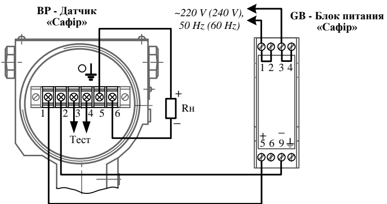
Рисунок В.2 - Схема соединений блока и одного датчика «Сафир» с выходным сигналом 0-5 (5-0) или 4 - 20 (20-4) мА по четырехпроводной линии связи
