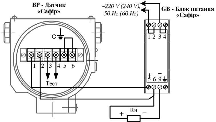
Рисунок В.1 - Схема соединений блока и одного датчика «Сафир» с выходным сигналом 4 - 20 (20-4) мА по двухпроводной линии связи
